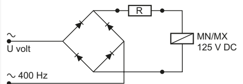
Wiring diagram.
